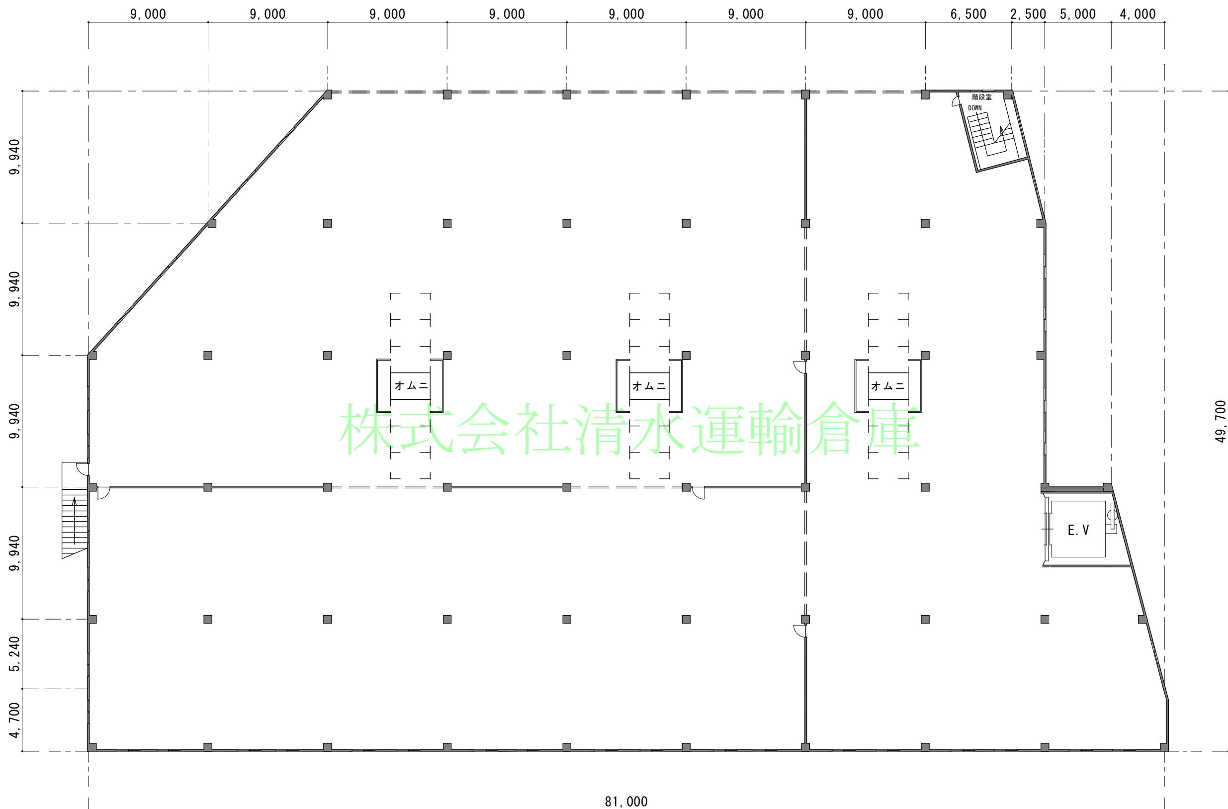
三ツ堀倉庫A棟 3F 平面図 S = 1 / 200
